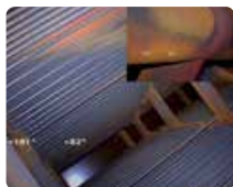
Alle Komponenten des Kondensators im Überblick und mit Zoom
