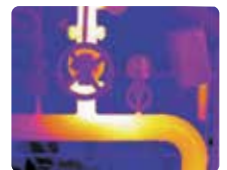
Thermografische Aufnahme einer defekten Absperrvorrichtung
